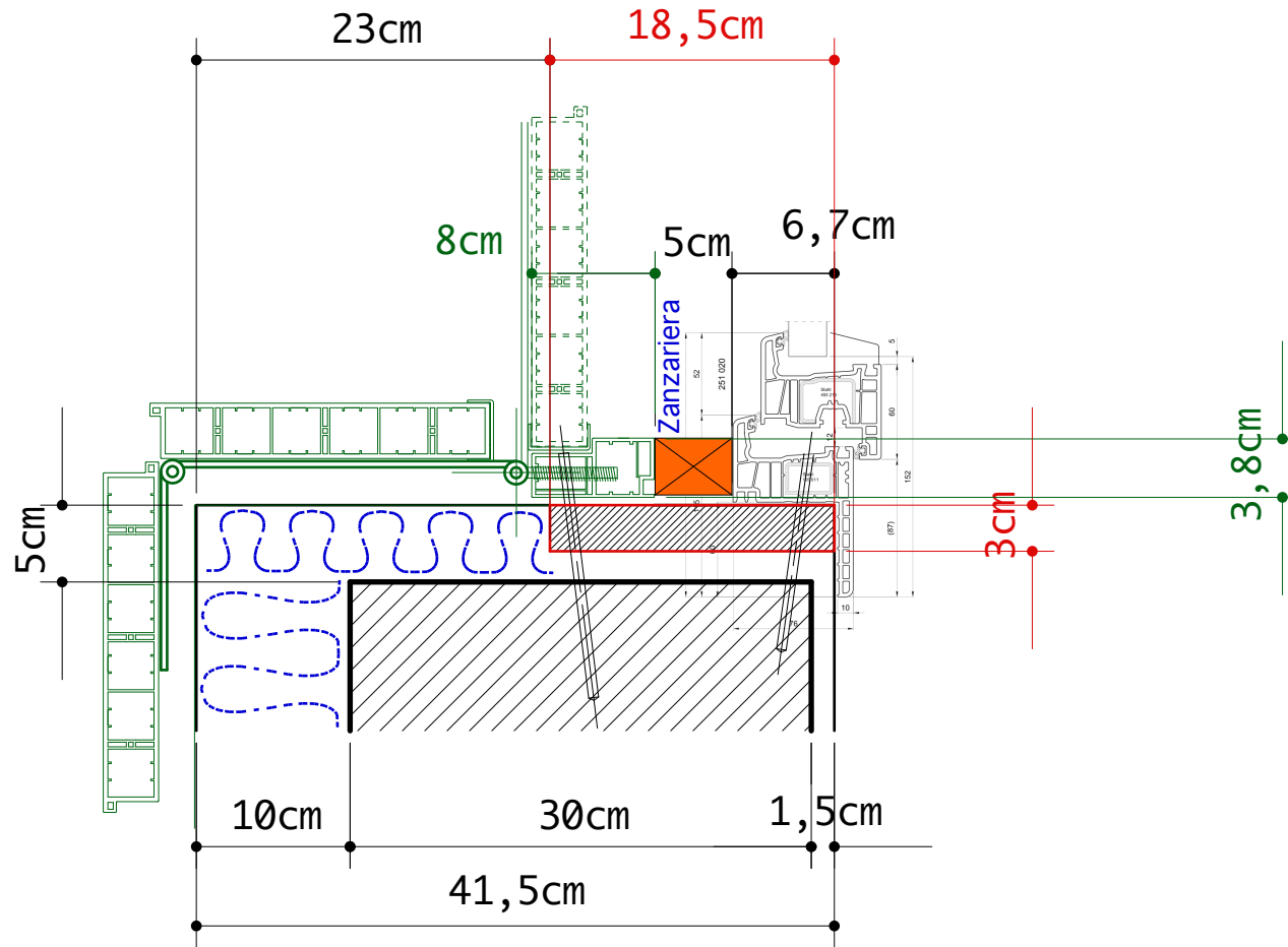
FINESTRA - ZANZARIERA - SCURO CON MONOBLOCCO
